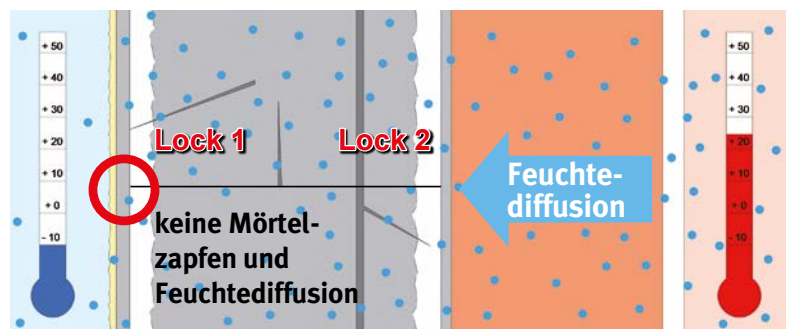
Plattenstosslösung Autolock DUOflex
